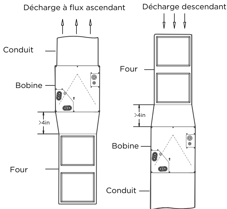
Installation Verticale à Débit Ascendant & Descendant
