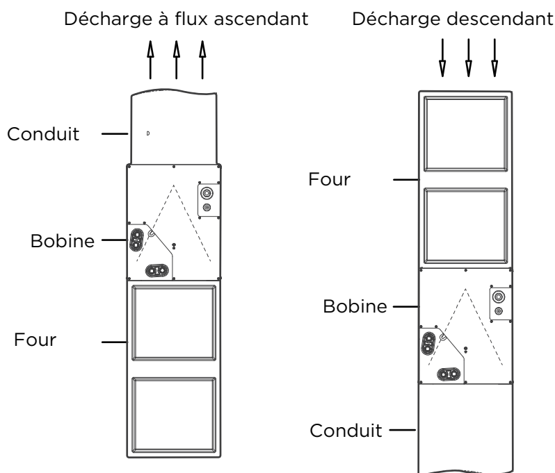
Installation Verticale à Débit Ascendant & Descendant
