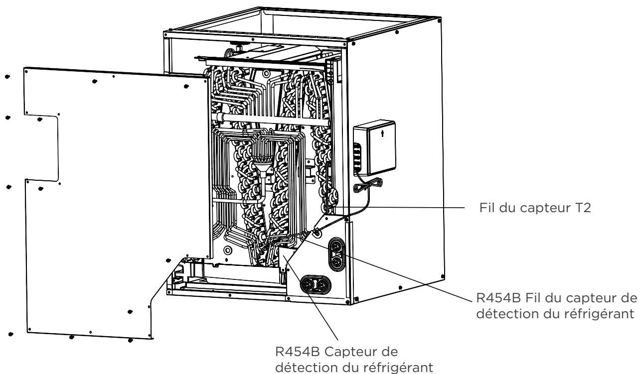
DIMENSIONS DU BOÎTIER ET EMBLACEMENT DES COMPOSANTS
