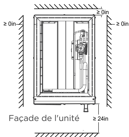
Vue en haut de l'écart de l'unité intérieure (y compris le conduit d'air)
