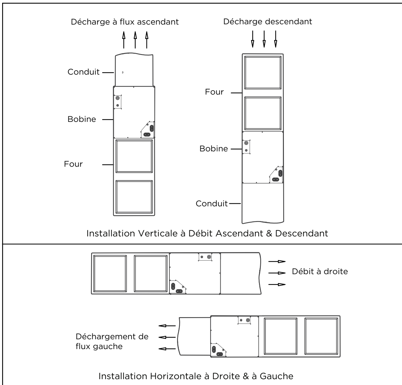
Type d'installation 2 : Modèle SENDC-60CO-C installation de la bobine sur le four
