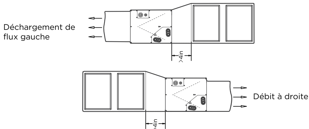
Installation Horizontale à Droite & à Gauche
